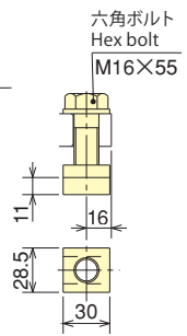
クランプ器具 Clamping Parts
