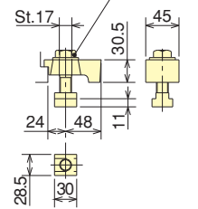
クランプ器具 Clamping Parts
